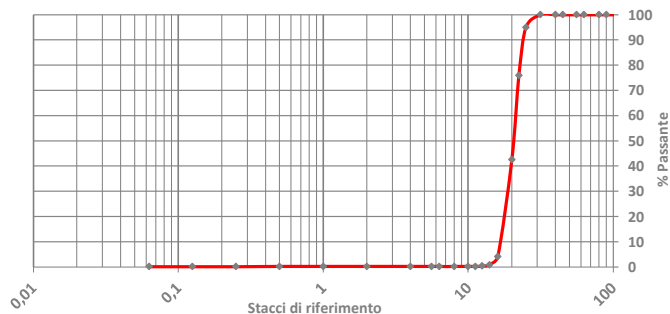
DoP N°3 - FT.CPR 305/2011 Curva Granulometrica Tipica - Carta Semilogaritmica
